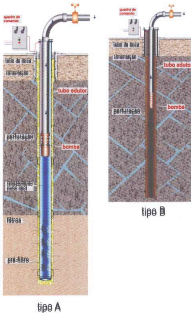
FIGURA 5- 8: PERFIS ESQUEMÁTICOS TÍPICOS DOS POÇOS
