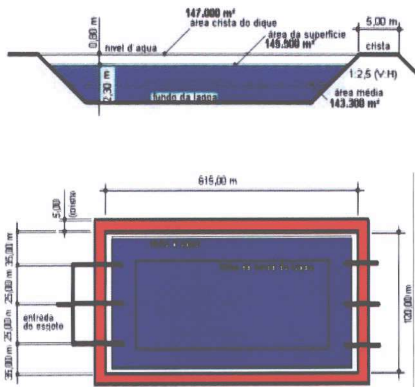
FIGURA 6- 7: LAGOA FACULTATIVA – SEÇÃO VERTICAL E PLANTA (SEM ESCALA)
