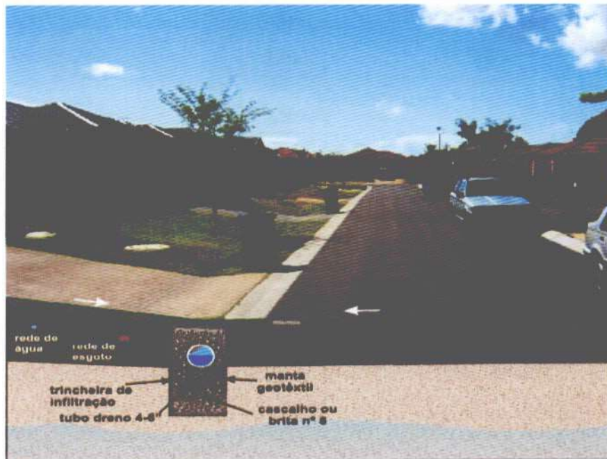
FIGURA 15- 6: SISTEMA DE DRENAGEM SUPERFICIAL E INFILTRAÇÃO NA CALÇADA – WSUD
