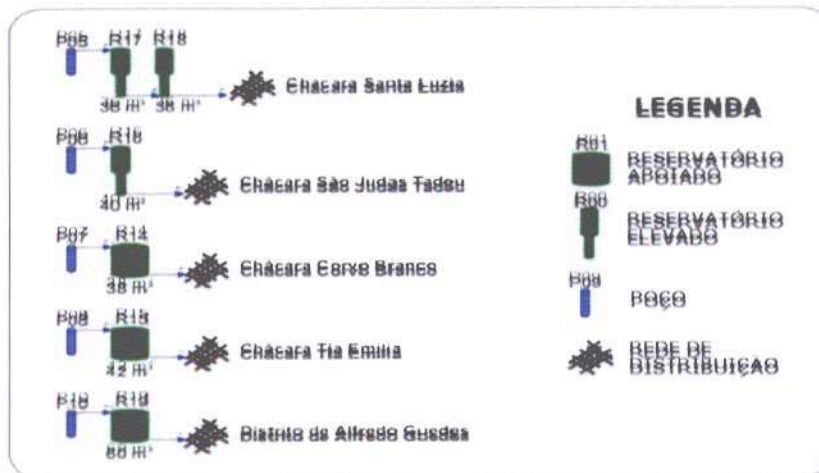
FIGURA 5- 10: REPRESENTAÇÃO ESQUEMÁTICA DOS SAA ISOLADOS
