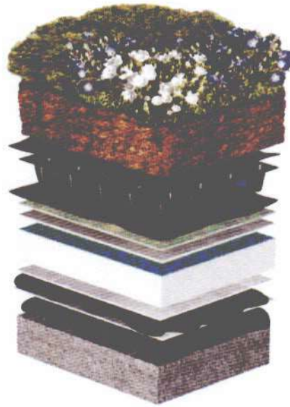
FIGURA 15- 17: ESQUEMA CONSTRUTIVO DE TELHADO VERDE (TELHADO VIVO)
